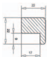
Type 80, standaard
